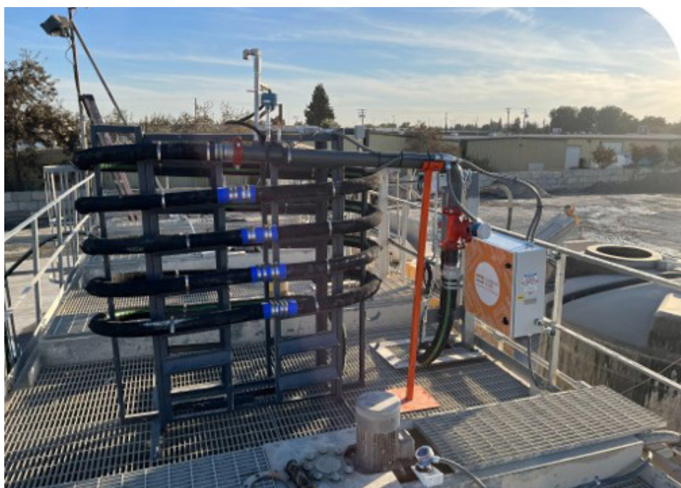
Installation du procédé CarbonCure pour le recyclage et la réutilisation des eaux usées. ©EDILTECO
